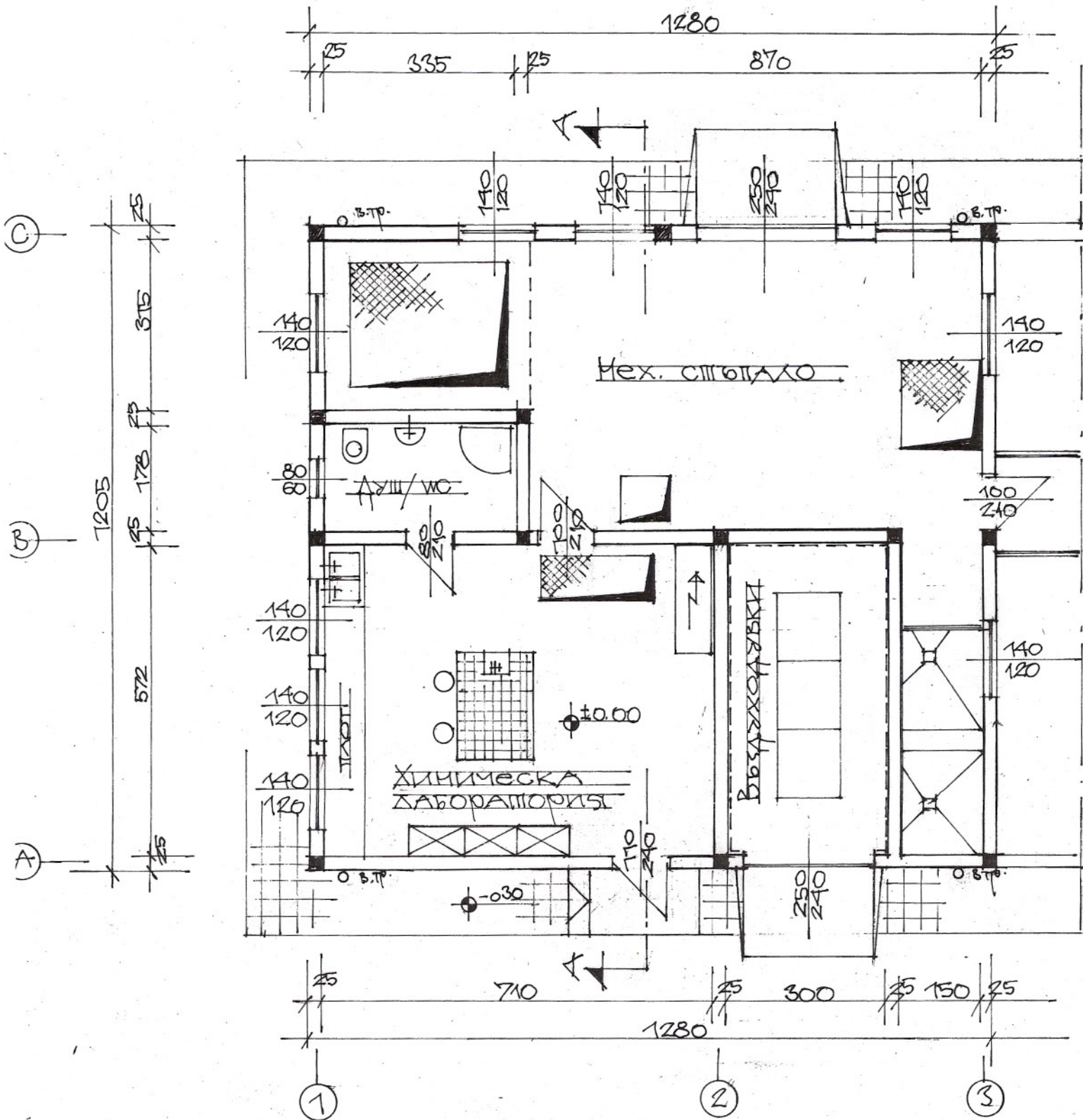
ПЛАН. М 1:100.
